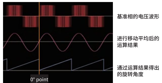
PWM 波形和旋转角度的记录示意图
